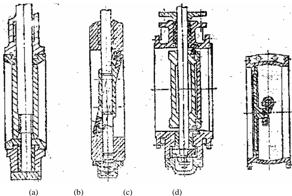
图 1-2 蝶阀结构图
